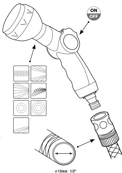
7F, SPRAY GUN WITH HOSE CONNECTOR – 1/2" PISTOLET NAWADNIAJĄCY 7F , Z SZYBKOZŁĄCZKĄ – 1/2"
