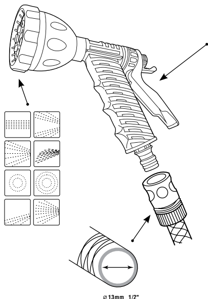
8F , SPRAY GUN WITH A SET OF QUICK CONNECT PIECES – 1/2" PISTOLET NAWADNIAJĄCY 8F , Z KPL. SZYBKOZŁĄCZY – 1/2"
