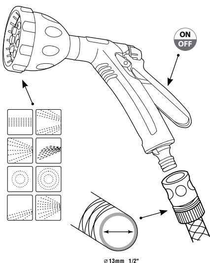
8F , SPRAY GUN WITH A SET OF QUICK CONNECT PIECES – 1/2" PISTOLET NAWADNIAJĄCY 8F , Z KPL. SZYBKOZŁĄCZY – 1/2"
