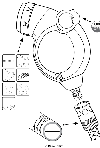
7F, SPRAY GUN WITH HOSE CONNECTOR – 1/2" PISTOLET NAWADNIAJĄCY 7F, Z SZYBKOZŁĄCZKĄ – 1/2"
