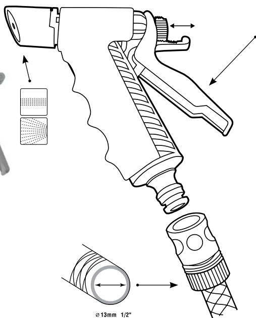
2F , SPRAY GUN WITH A SET OF QUICK CONNECT PIECES – 1/2" PISTOLET NAWADNIAJĄCY 2F , Z KPL. SZYBKOZŁĄCZY
